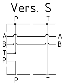
collegamento serie series connection
