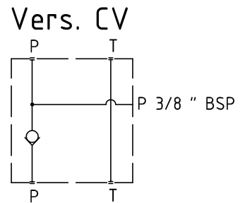
ritegno su P check valve on P
