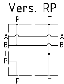
per valvola riduttrice for reducing valve
